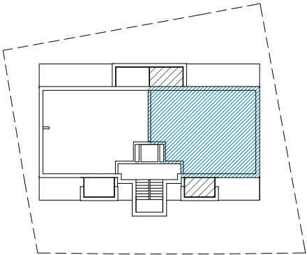
2.DACHGESCHOSS
